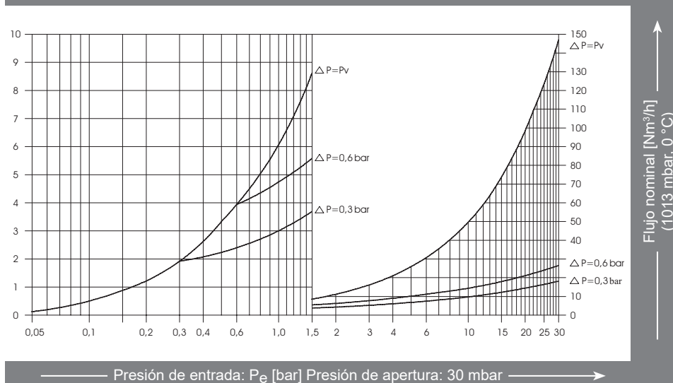
Diagrama de flujo para aire (20 °C)
