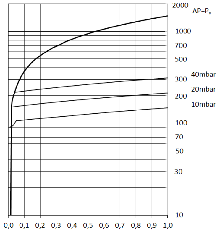
Diagram przepływu powietrza (20 °C)
