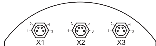
vorgeschriebene Einbaulage bei Auswahl der Modellvariante mit „Flow“
